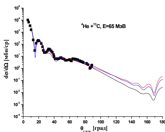
2 сурет – 26.6 және 65 МэВ аралығында альфа-бөлшектердің {}^{13}\text{C} ядроларынан серпімді шашыруының дифференциалдық қималары. Көк түспен көрсетілген қисық сызықтар оптикалық модель нәтижесінің А жинағы, 29 және 65 МэВ энергиялар үшін В жинағы қара түсті қисық сызықтармен көрсетілген. Қызыл түсті қисық сызықтар фолдинг моделі бойынша есептеу нәтижелері
