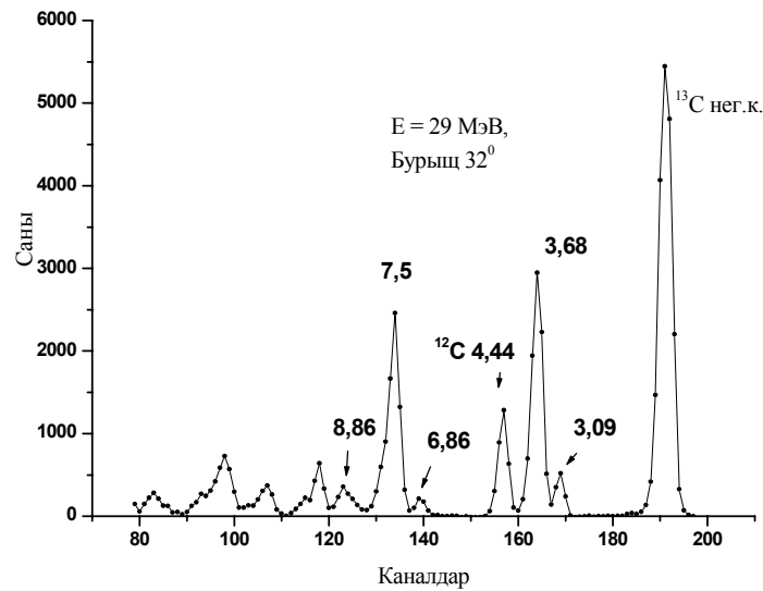
1-сурет – альфа-бөлшектердің ^{13}\text{C} ядроларында E=29 МэВ энергияда шашырауының энергетикалық спектрі ( 32^\circ )
