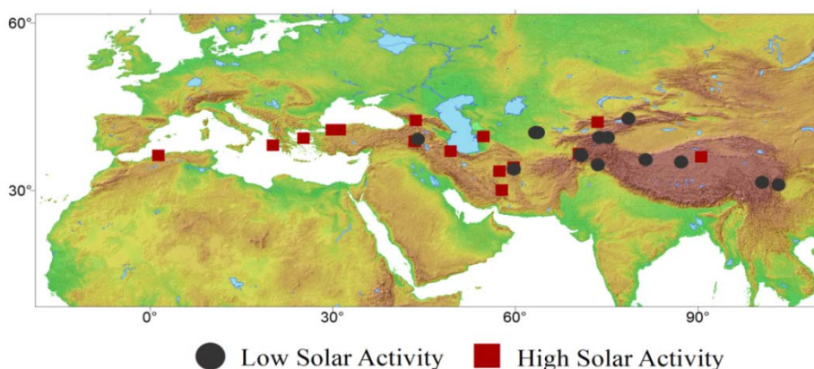
Рисунок 2 – Распределение эпицентров сильных землетрясений ( M \geq 7.0 ), произошедших в 1973-2014гг на территории с координатами 30^{\circ}N-45^{\circ}N, 0^{\circ}E-110^{\circ}E : черные круги – эпицентры событий, произошедших при пониженной солнечной активности, красные квадраты – при повышенной солнечной активности.
